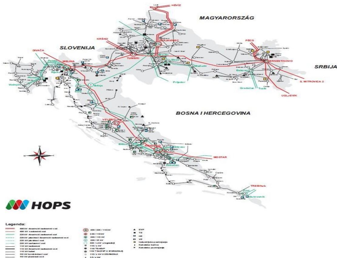
Slika 5. Elektroenergetska mreža Republike Hrvatske u 2015. godini
