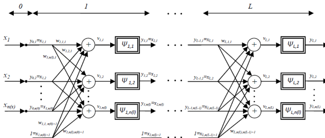
Slika 2.8: Višeslojna perceptronska mreža (MLP mreža). [23]
