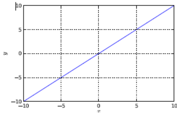
Slika 2.4: Linearna funkcija [9]
