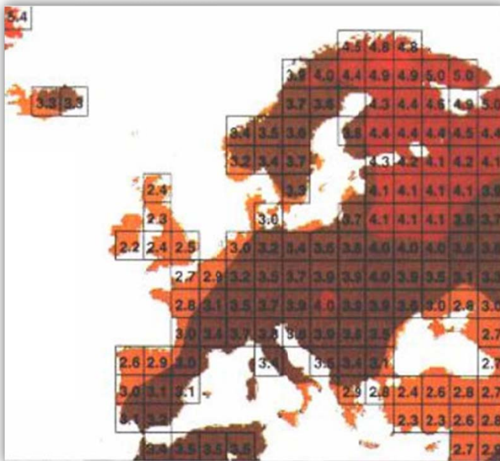
Slika 12. Mogući scenarij porasta temperature do 2050. godine.
