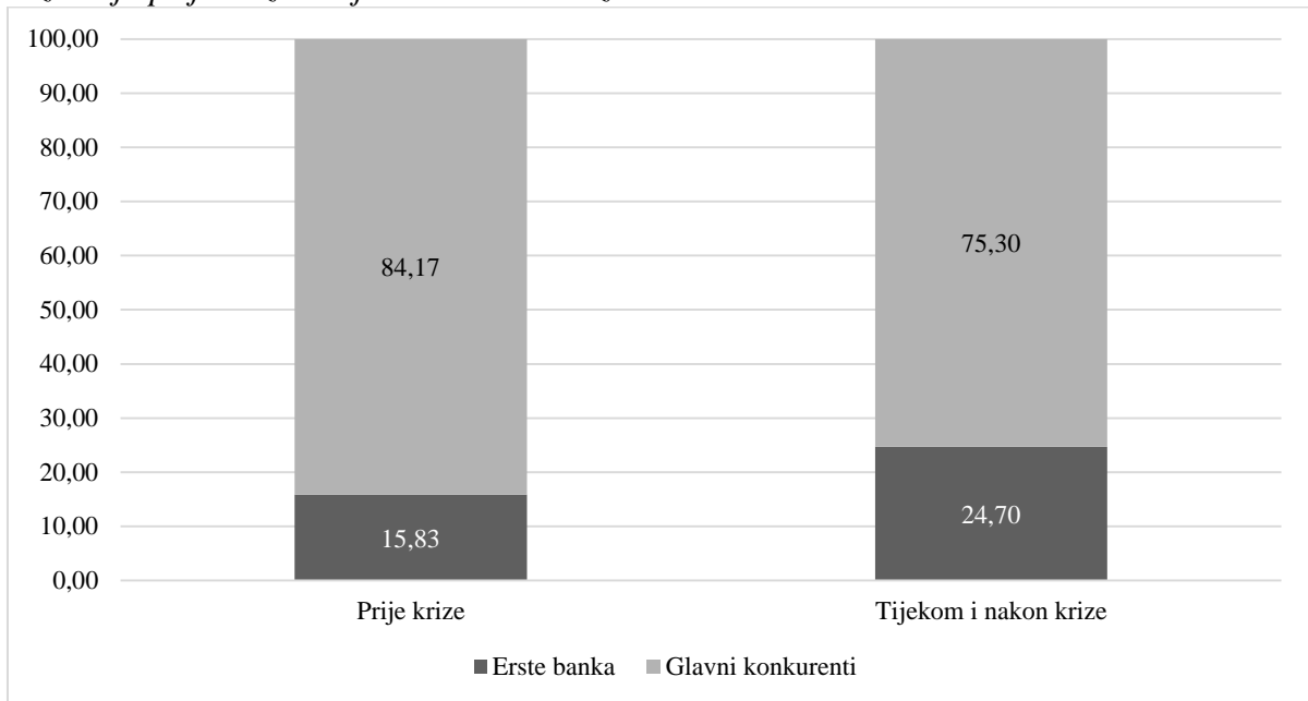
Grafikon 2: Prosječno stanje udjela aktive Erste banke u odnosu na glavne konkurente u razdoblju prije krize te tijekom i nakon krize
