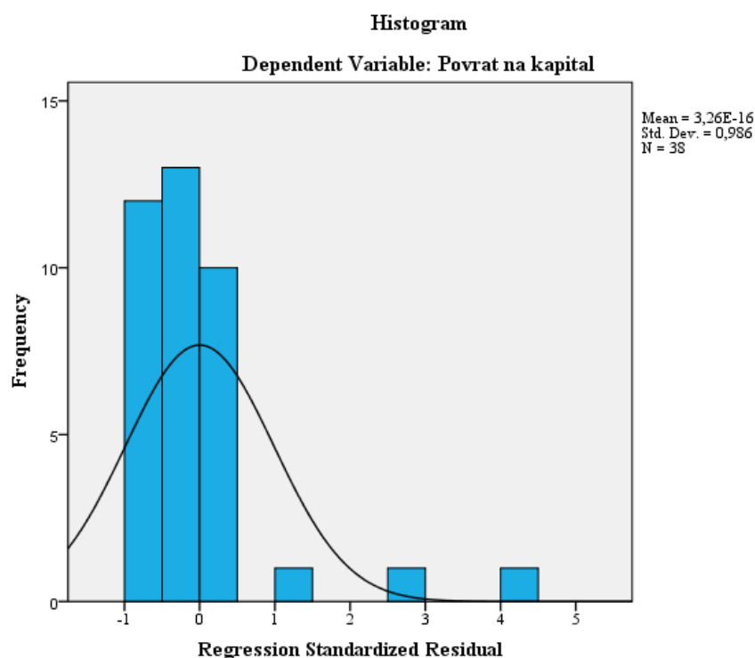
Graf 10: Histogram standardiziranih reziduala (H3)
