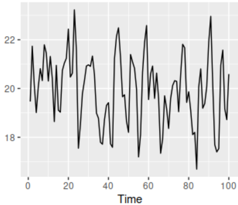
Slika 5 - Model MA(2)
