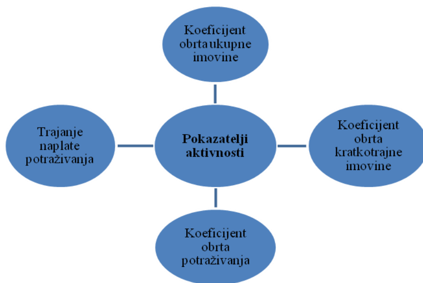
Slika 7: Pokazatelji aktivnosti
