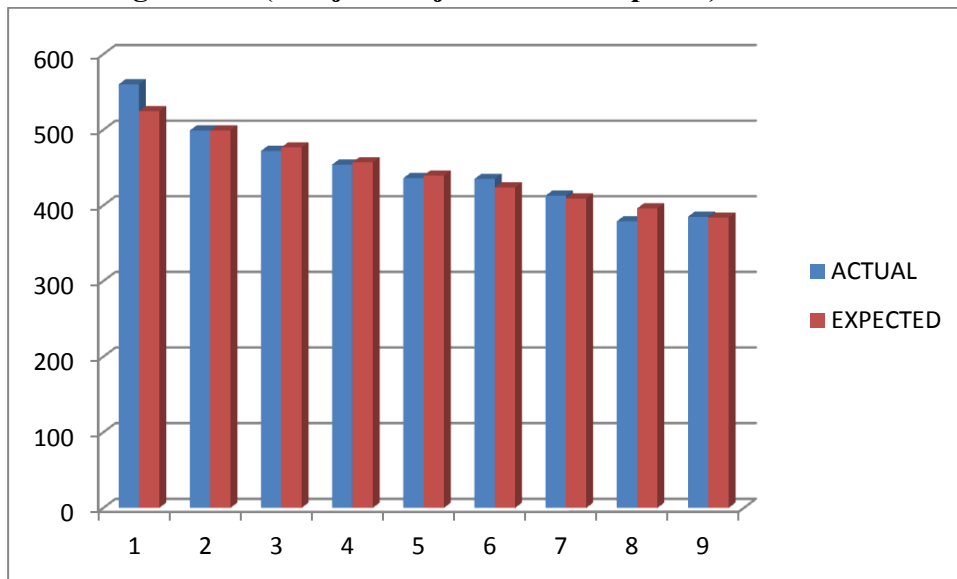
Grafikon 12: Stvarne i očekivane frekvencije znamenke na drugoj brojevnoj poziciji u iznosima gubitaka (manje razvijena tržišta kapitala)
