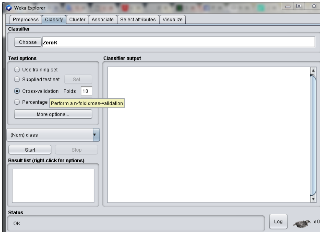
Slika 18. prozor 'Classify'
