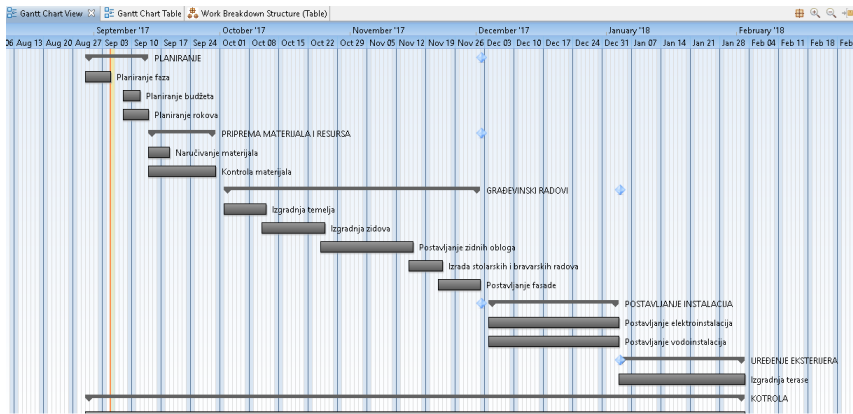
Slika 9. Gantt Chart
