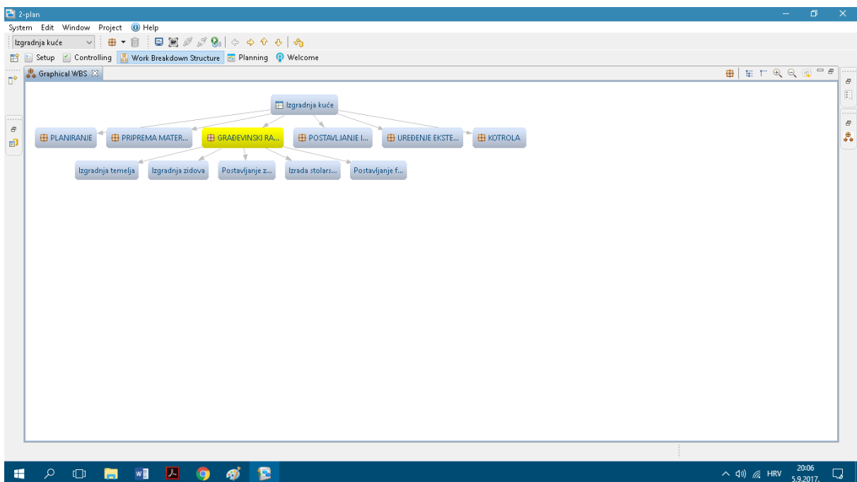
Slika 8. Grafički WBS
