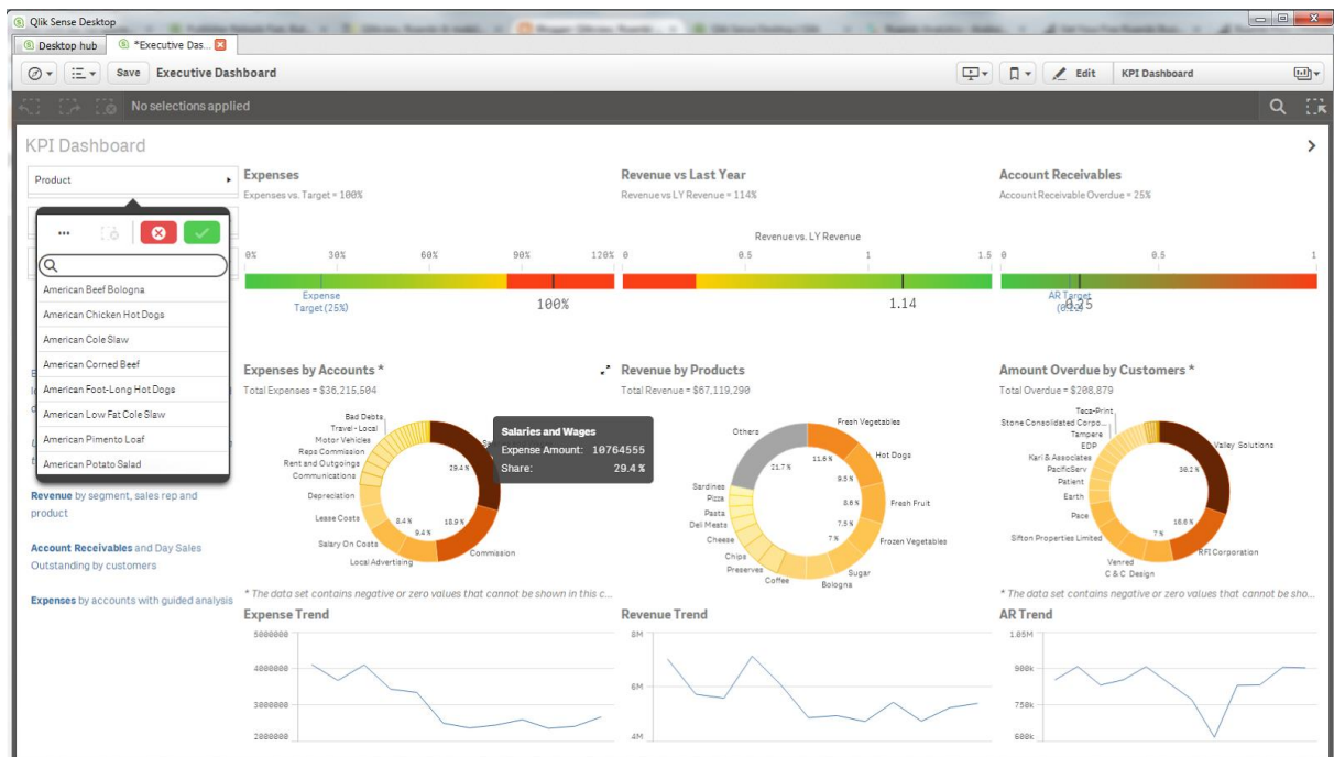
Slika 9. QlikSense dashboard
