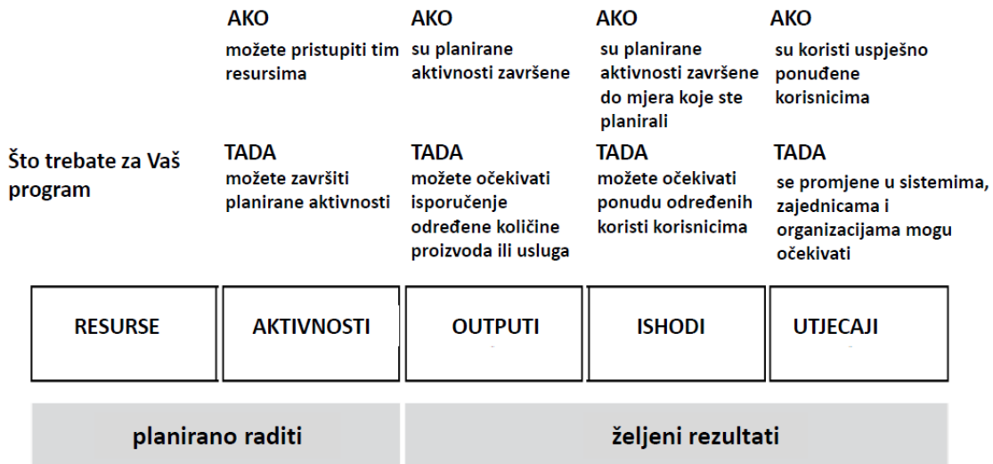
Slika 7. Logički model
