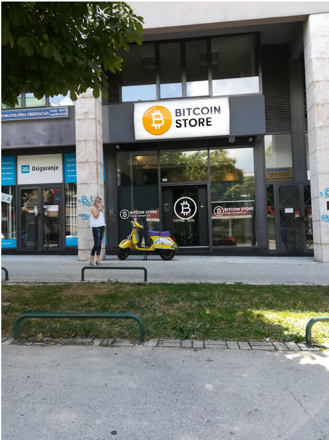
Slika 3. Bitcoin mjenjačnica
