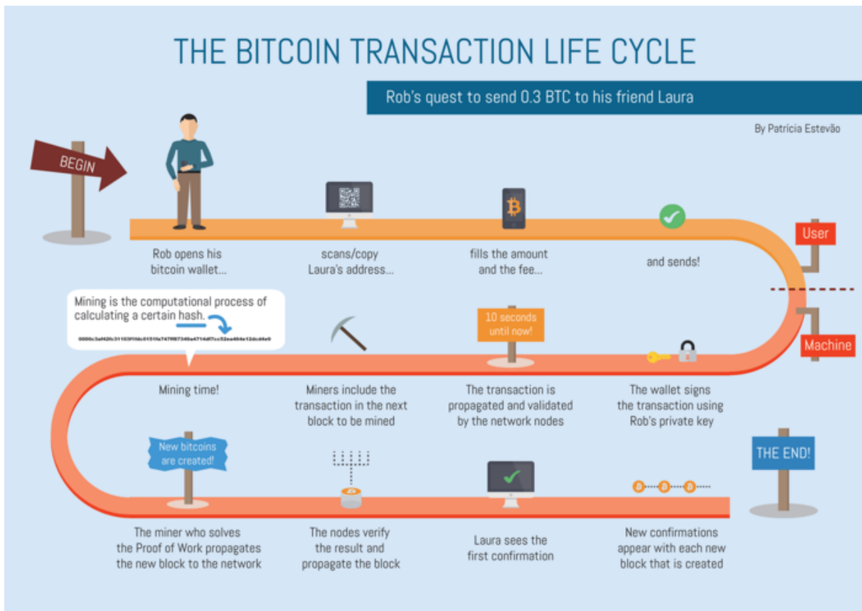
Slika 2. Bitcoin transakcija
