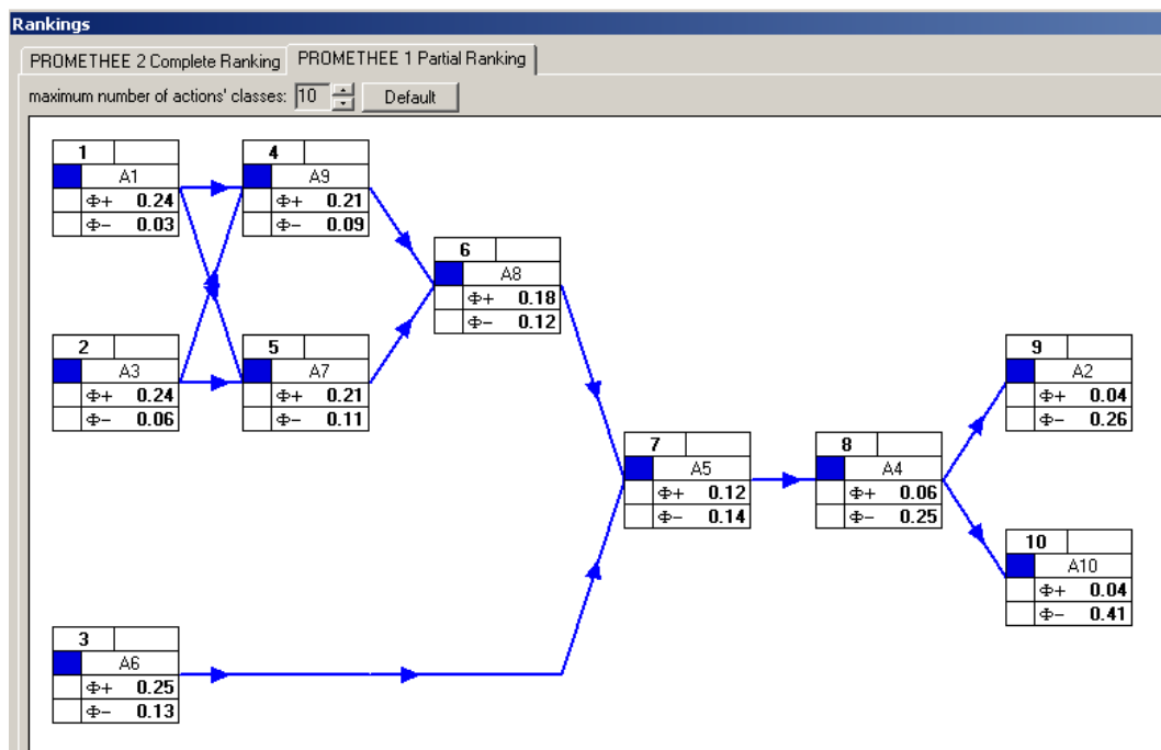
Slika 12. PROMETHEE I – parcijalni uredaj
