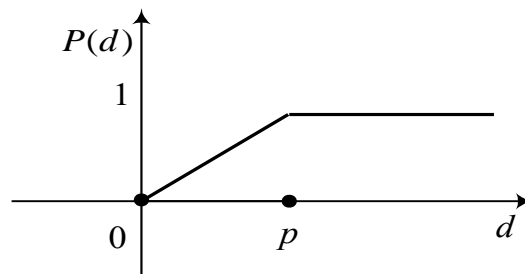
Slika 6. Kriterij s linearnom preferencijom
