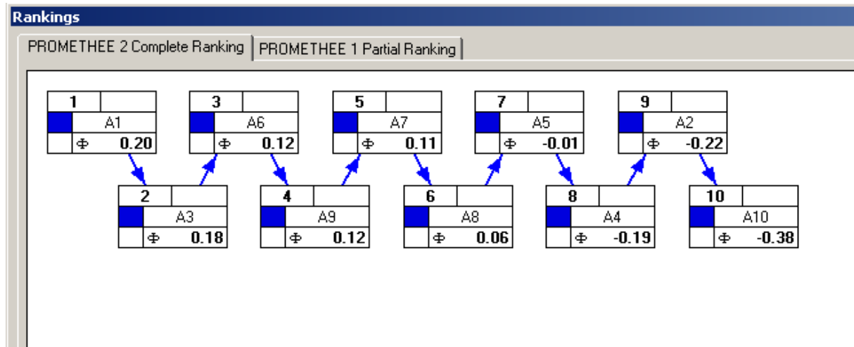
Slika 13. PROMETHEE II-Kompletni poredak
