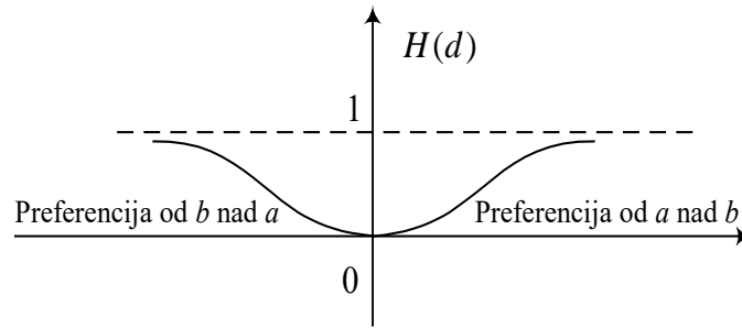
Slika 3. Funkcija preferencije H(d)
