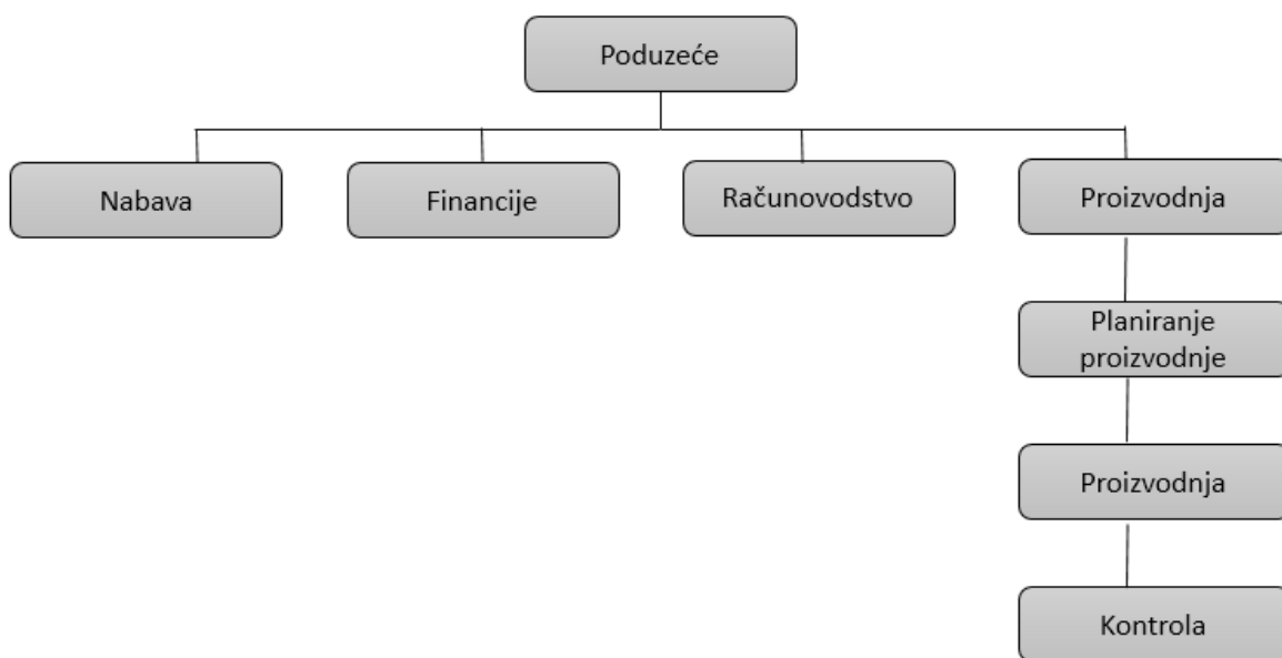
Slika 3: WBS organizacije
