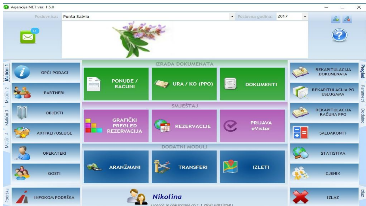
Slika 6. Agencija.NET aplikacija
