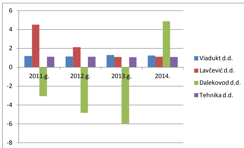
Graf 8: Prikaz pokrivanja troškova kamata
