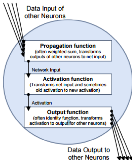
Slika 9. Obrada informacija u neuronskoj mreži izvor: ( http://eris.foi.hr/11neuronske/nn-predavanje4.html )
